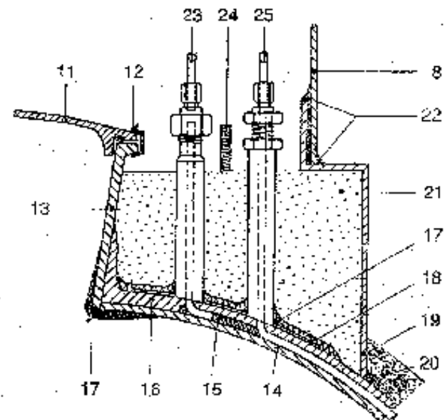
Détail A
